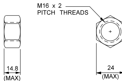
NUT DETAILS 1:2
